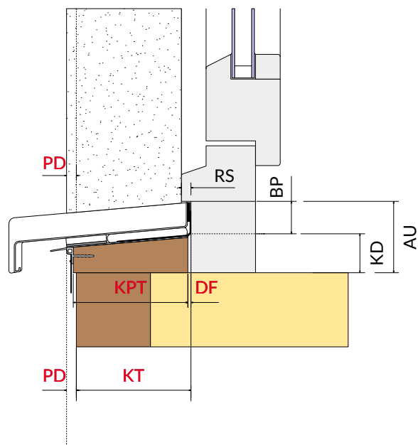
Vertikalschnitt Fenster B - B
