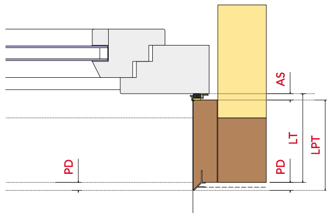
Horizontalschnitt Fenster A - A
